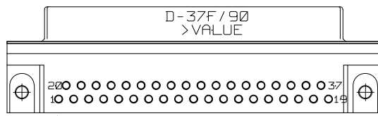
D-37M
