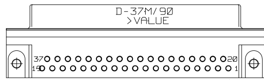
D-37F
