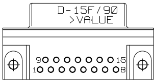
D-15F
