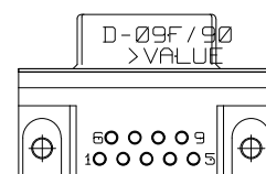
D-09F
